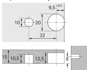
Esquema de furação
